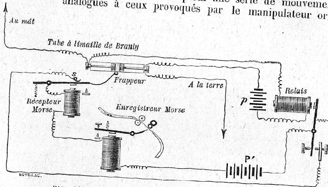
FIG. 140. — RÉCEPTEUR DE TÉLÉGRAPHE SANS FIL.
