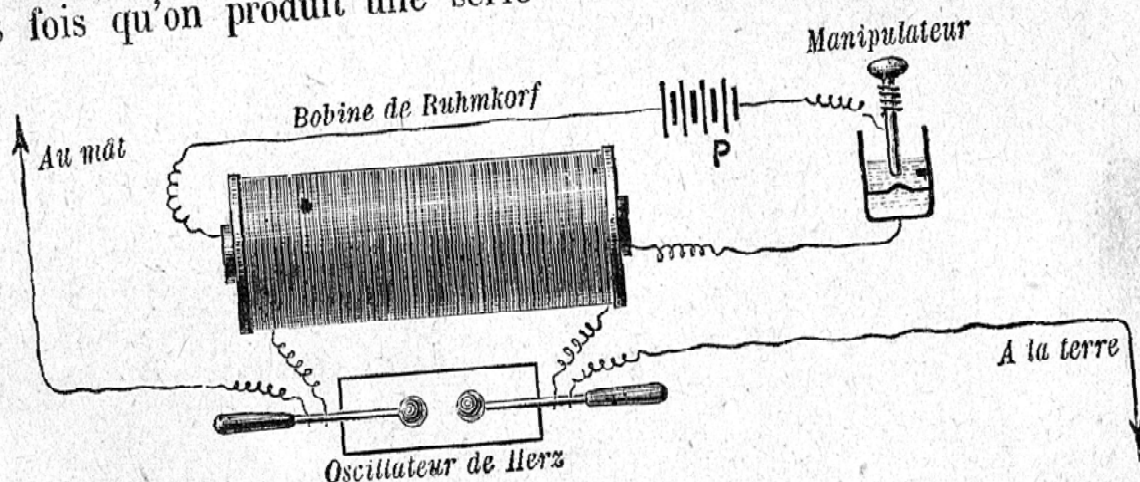
FIG. 139 bis. — TRANSMETTEUR DU TÉLÉGRAPHE SANS FIL.
