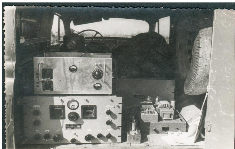
Récepteur Hammarlund + constructions OM
